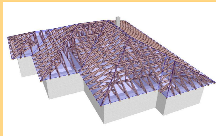
Tetőszerkezet
